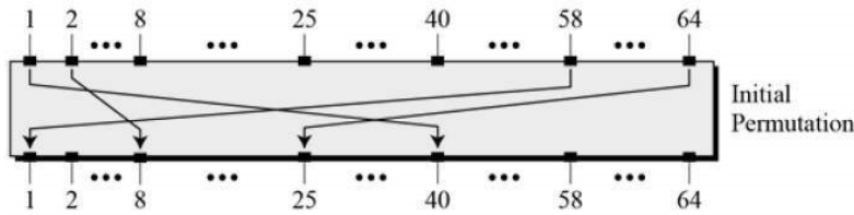
Рис. 2 Початкова перестановка
