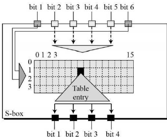
Рис. 8. Правило S-блоків
