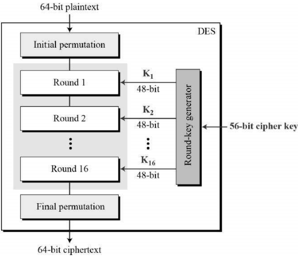
Рис. 1. Структура DES
